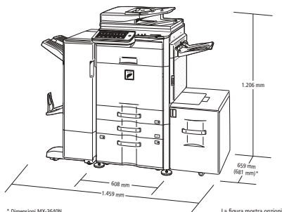
* Dimensioni MX-3640N
